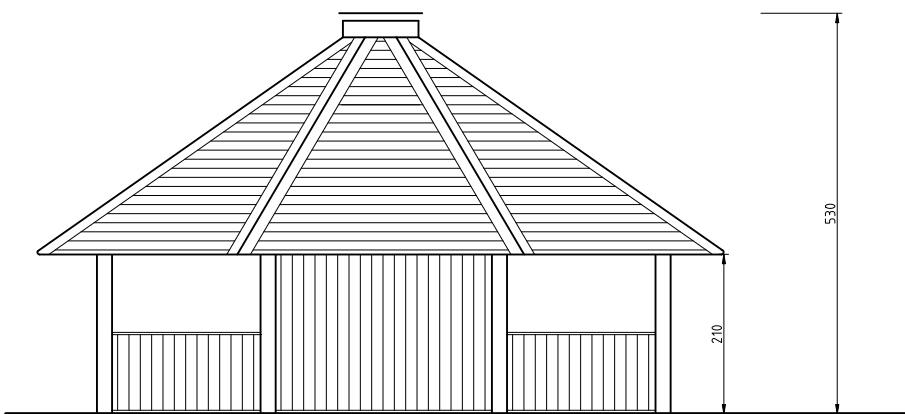
Facader, syd og vest
