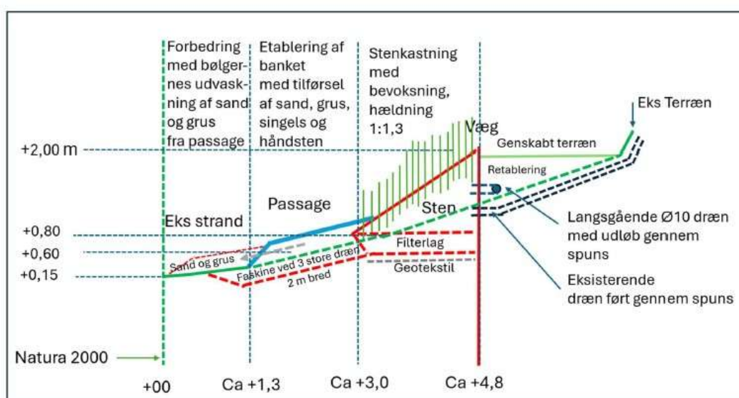
Figur 1b: principielt tværsnit af det ansøgte projekt, ansøgning af 22. oktober 2025
